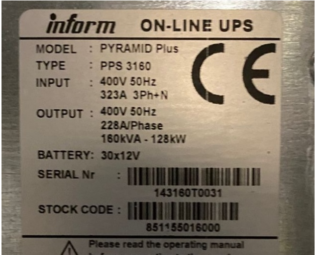
ACTUAL NAMEPLATE
